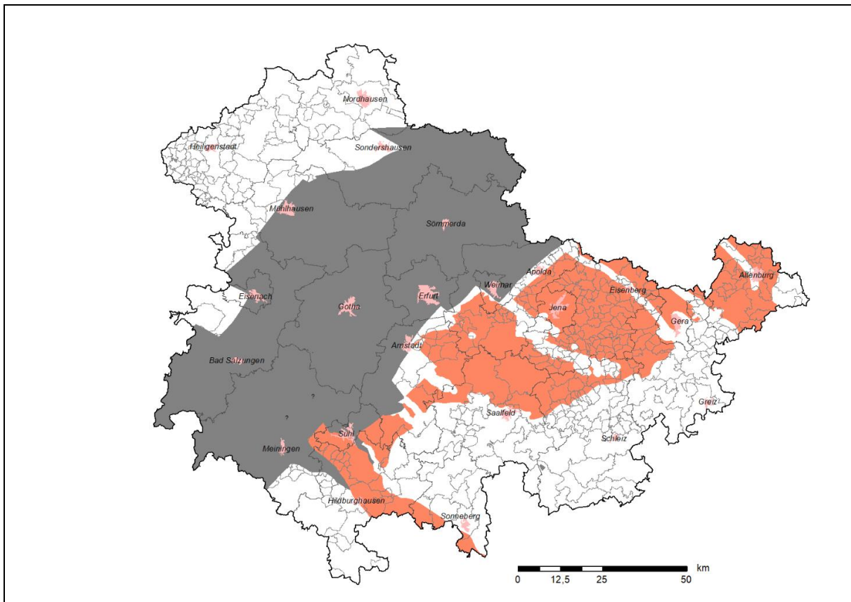
Abb. 6: Teilgebiet 009_00TG_194_00IG_K_g_SO (hellrot) und Verbreitung kristalliner Wirtsgesteine nach der Karte des tiefen Untergrundes in Thüringen (grau) (Erstellung TLUBN).
