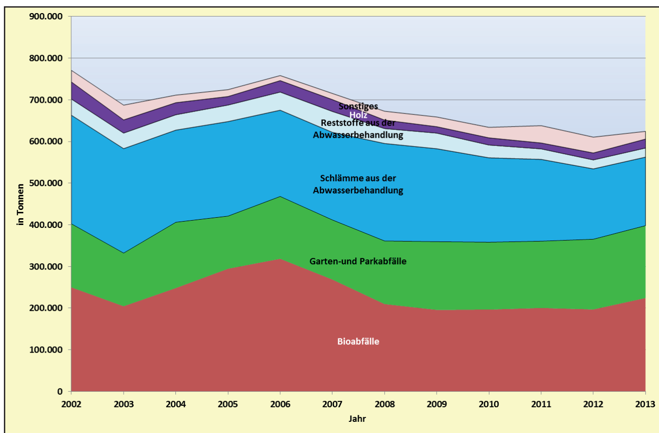
Abb. 3: In Kompostierungsanlagen angenommene Abfälle in Thüringen 2002 bis 2013, zusammengefasst in Abfalloberguppen
