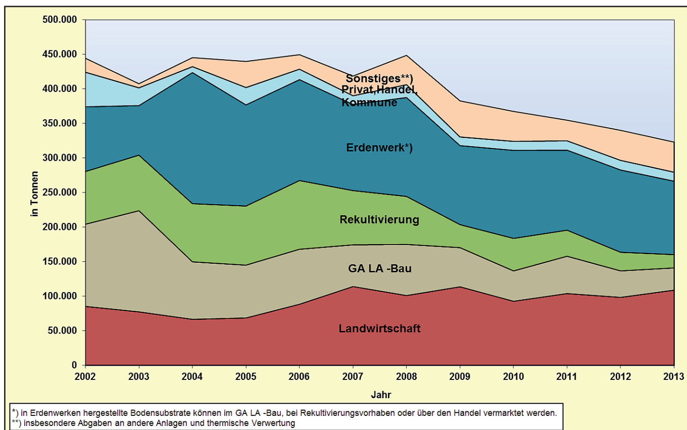
Abb. 5: Mengenentwicklung der Verwertungswege der erzeugten Komposte in Thüringen 2002 bis 2013
