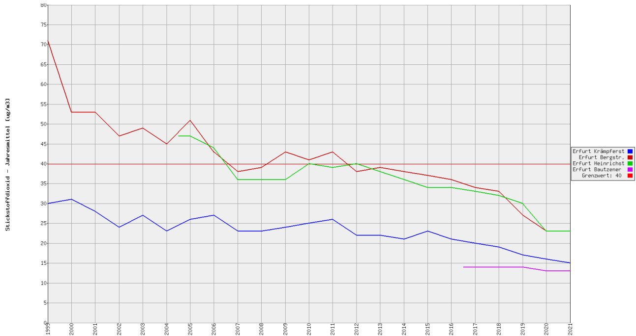
Abbildung 6: Entwicklung der NO 2 -Konzentrationen im Jahresmittel an den Messstationen in Erfurt
