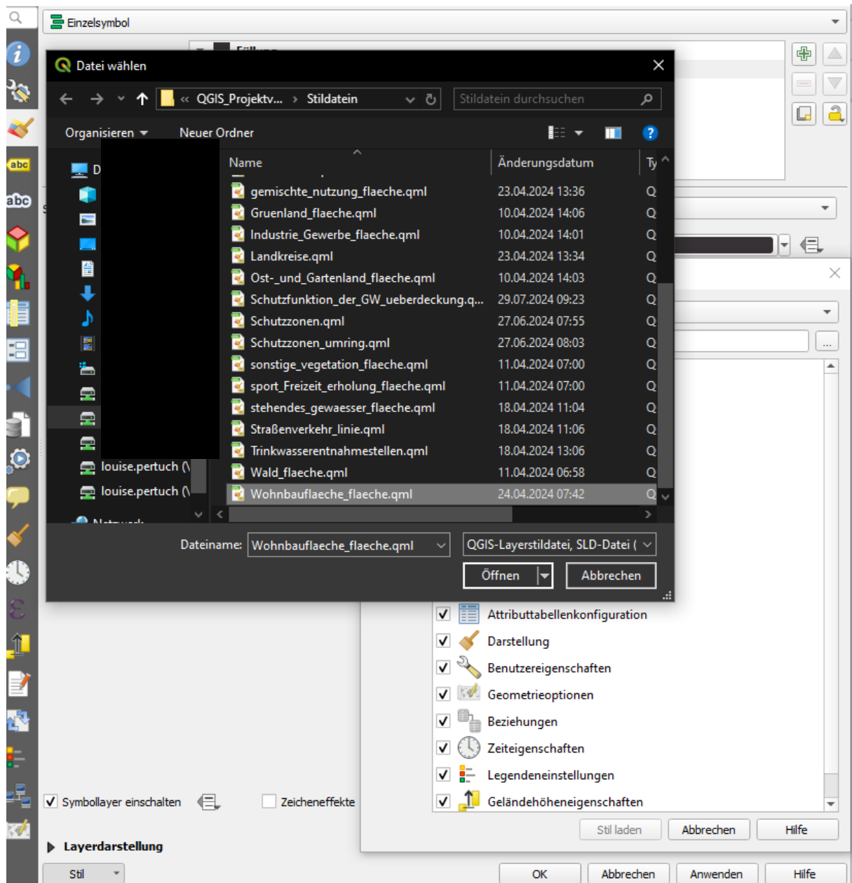
Abbildung 17 Stil auswählen
