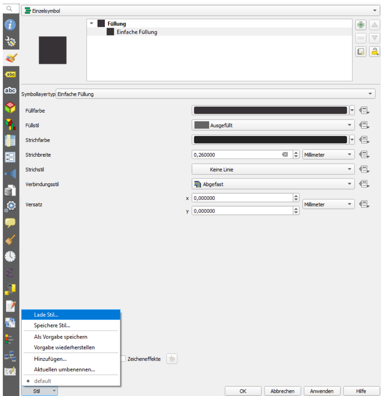
Abbildung 16 Stil laden
