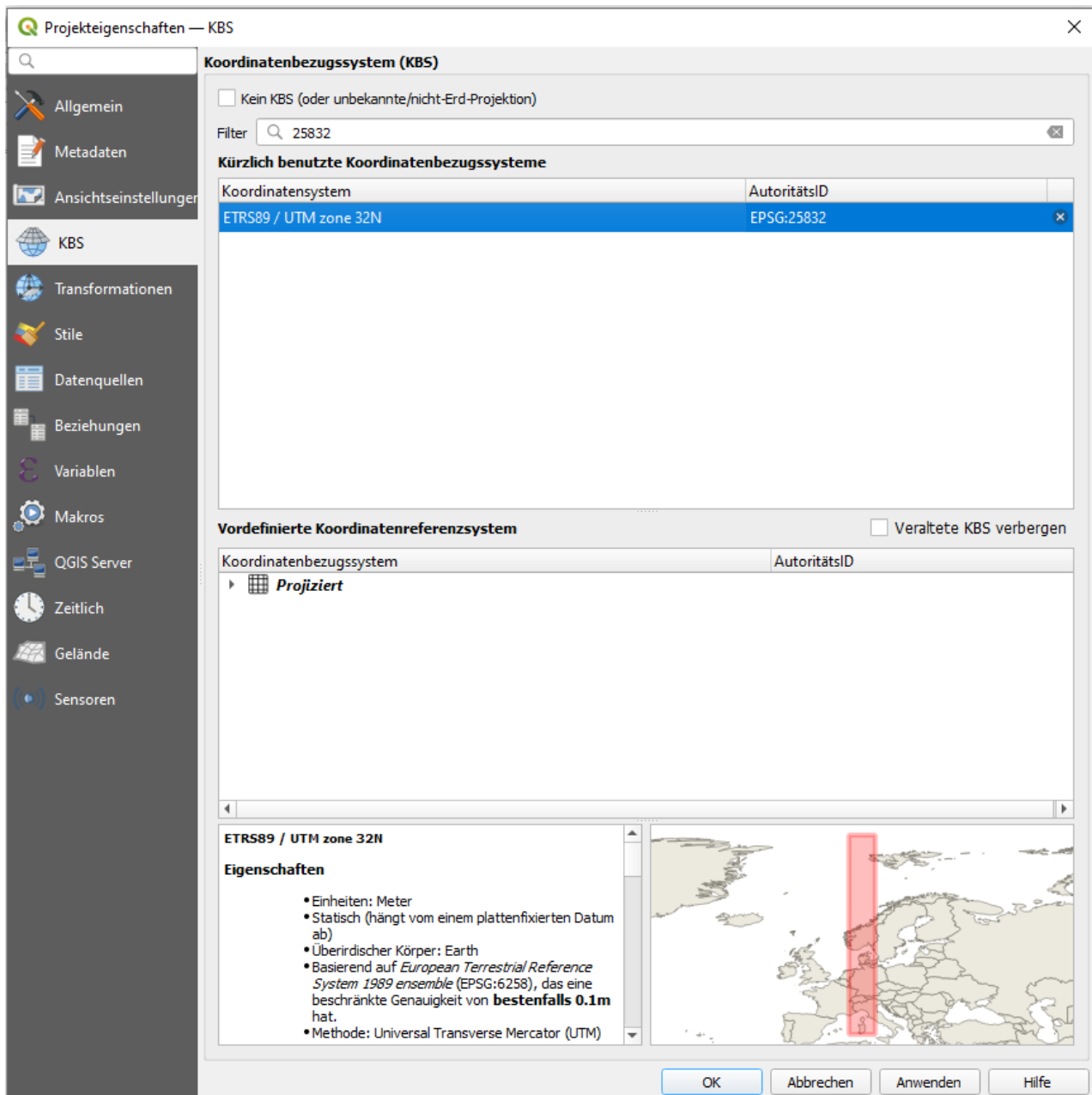
Abbildung 4 Koordinatenbezugssystem Auswahl
