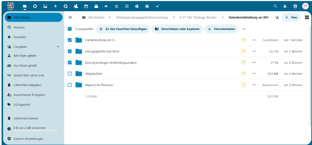
Abbildung 12 Downloadfenster ThDAP
