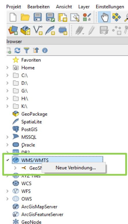
Abbildung 5 WMS Verbindung
