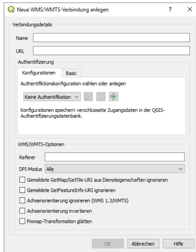
Abbildung 6 WMS Parameter
