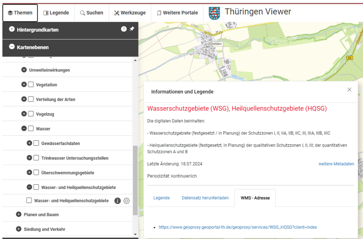
Abbildung 10 WMS Dienste
