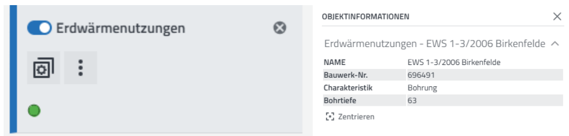
Abbildung 4 Objektinformation zu einer Erdwärmennutzung in Karte 6
